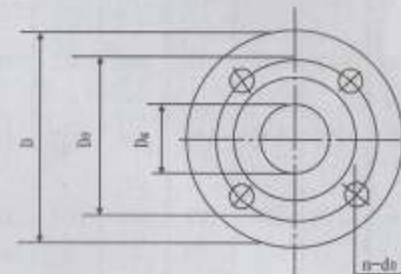
吸入吐出法兰
