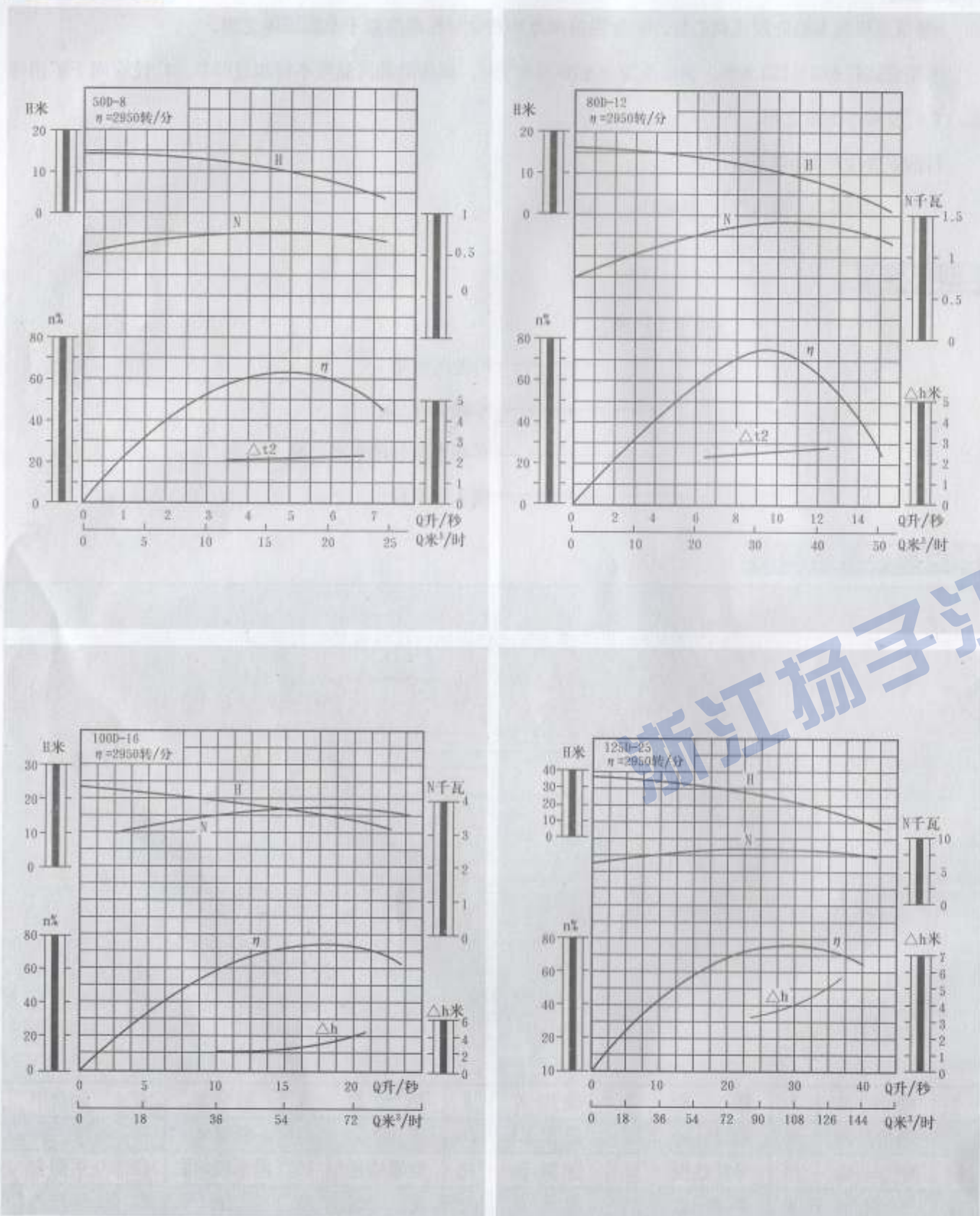
性能曲线图
