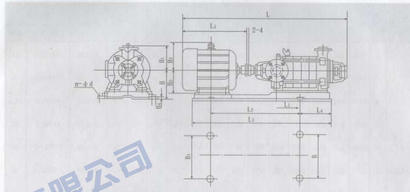
D型离心水泵外形尺寸
