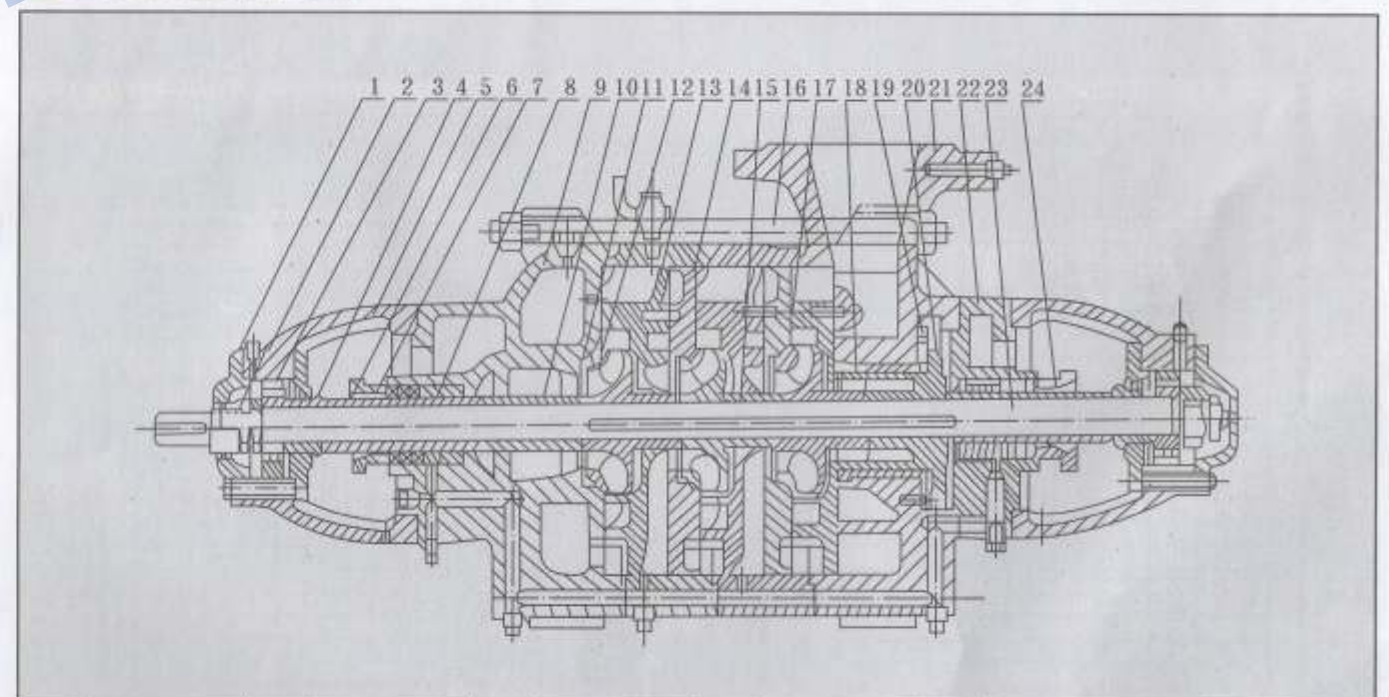
D型离心泵结构图
